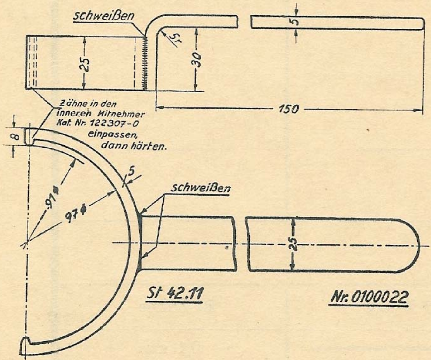
Halteschlüssel für inneren Mitnehmer der Kupplung sämtlicher NZ-Baumuster
