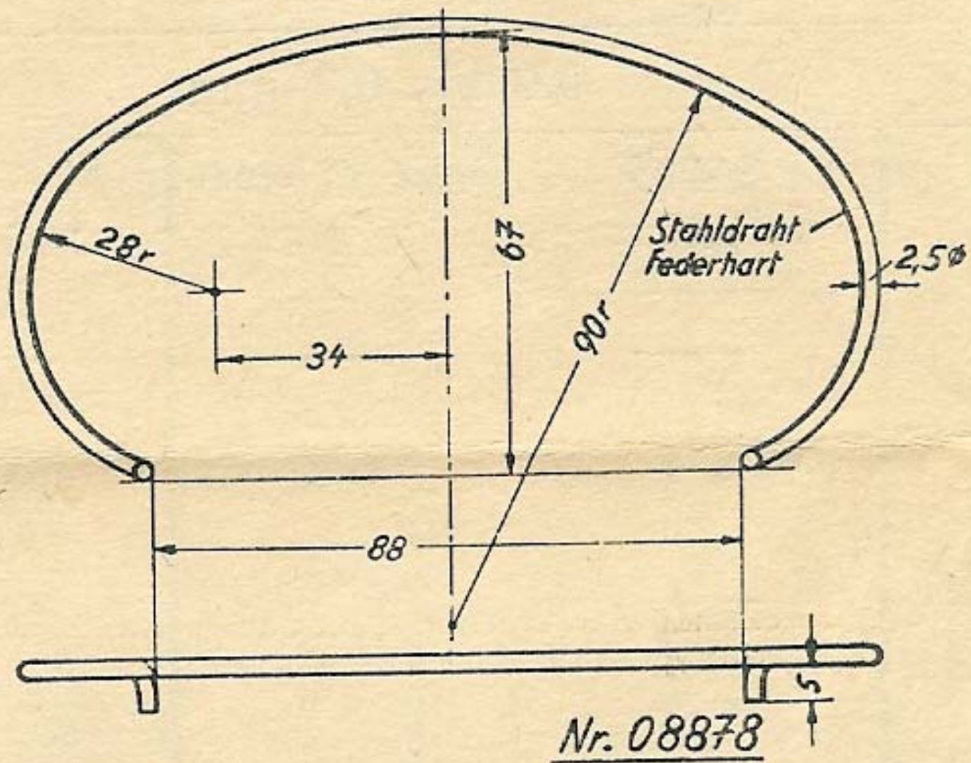
Fliehgewicht-Ausdrücker für Zünd- regler der Baumuster NZ 250 und NZ 350
